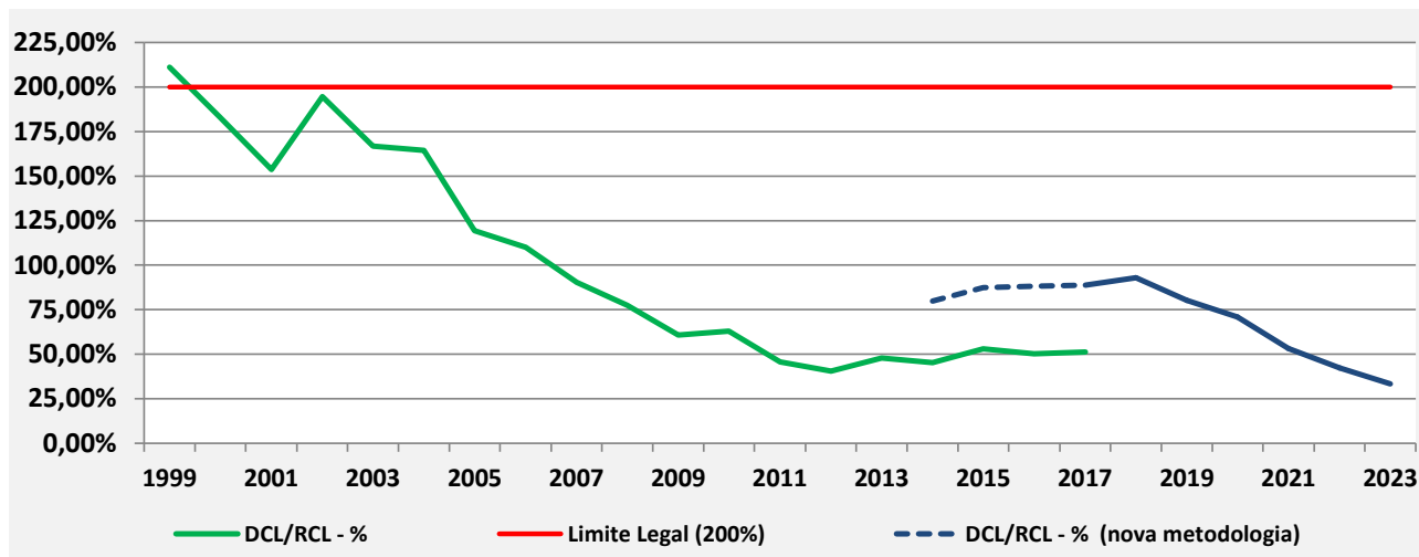
Gráfico 06 - % DCL/RCL – 1999 a 2023
