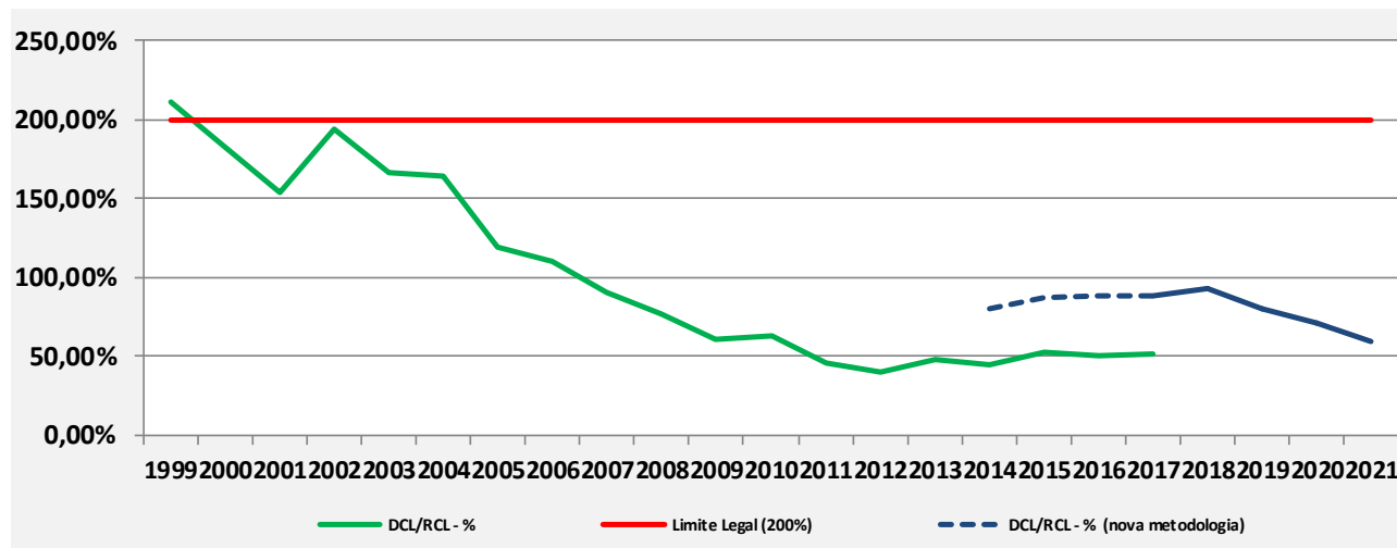
Gráfico 05 - % DCL/RCL – 1999 a 2021
